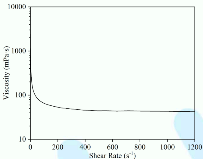
Fig 3 : 40°C剪切速率与黏度关系
